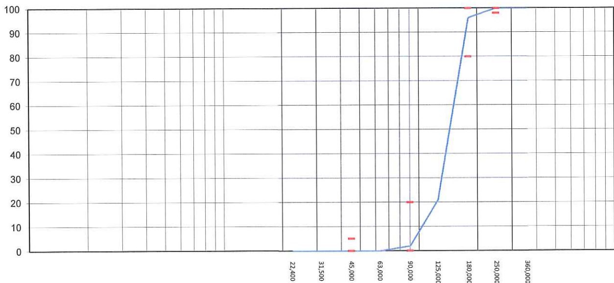
Curva Granulométrica Tipo
